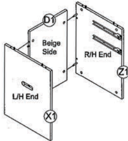
A. Insert Cam Bolt
